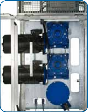
Grupo motriz: paracaídas de seguridad montado en piñón independiente, reductores con corona sin-fin y motor con electrofreno integrado Drive unit: overspeed emergency brake on a independent pinion and gearmotors with built-in electric brake
